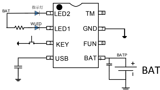
图一 QW2672K 典型应用电路
